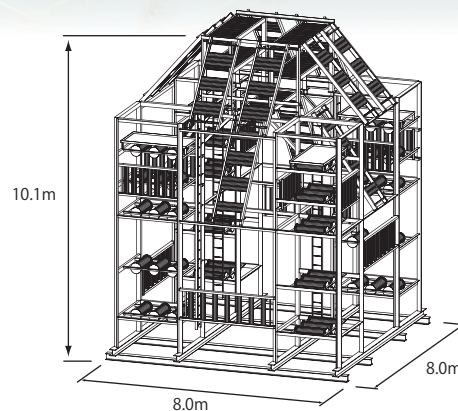
対象魚礁：シェルナース 10.0 型
