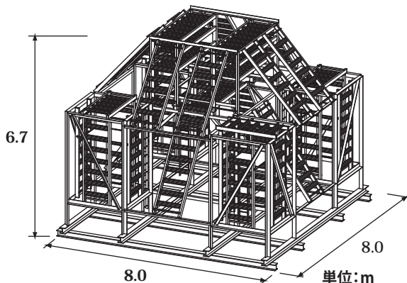
対象魚礁：シェルナース 6.0 型
