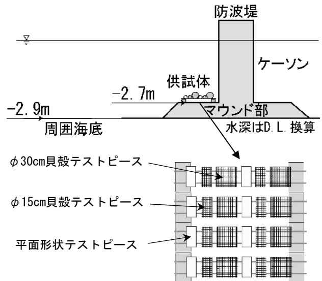
図-2 供試体の概略配置
