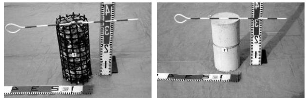
写真-2 テストピース（左：貝殻基質，右：コンクリート基質）
