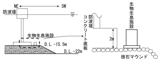
図-4 設置海域の断面および生物生息施設状況
