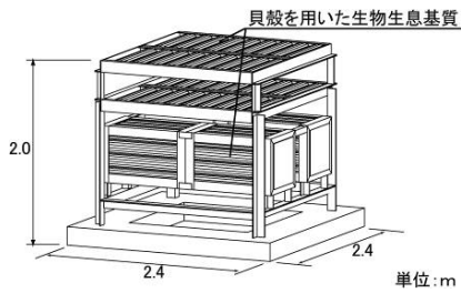
図-1 生物生息施設
